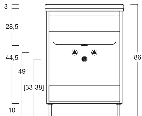
Misure interno vasca L 52 x P 29 x H 26 Su richiesta: Strizzatoio in legno ART.400AX
